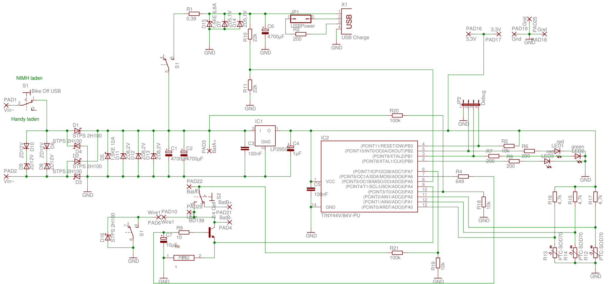
Fahrradlader (c) 2012 Malte Marwedel
